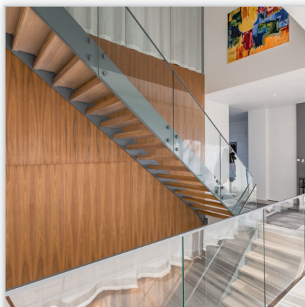
Schody STAVANGER – konstrukcja ze stali malowanej proszkowo, stopnie dębowe, balustrada szklana FLAT.
